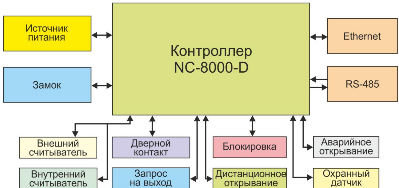
Рисунок 5. Оборудование, подключаемое к контроллеру NC-8000-D
