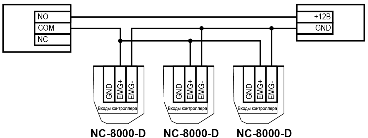
Рисунок 19. Схема подключения одной аварийной кнопки к нескольким контроллерам
