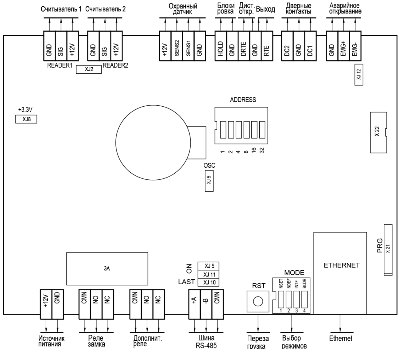
Рисунок 3. Схема платы контроллера NC-8000-D
